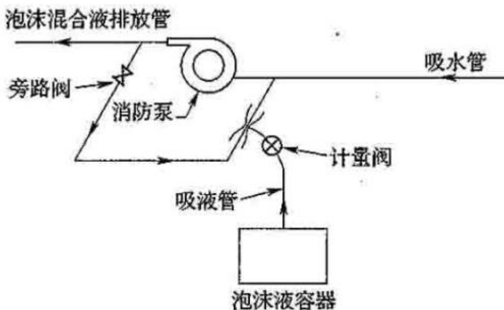
图 2 环泵式比例混合流程示意
