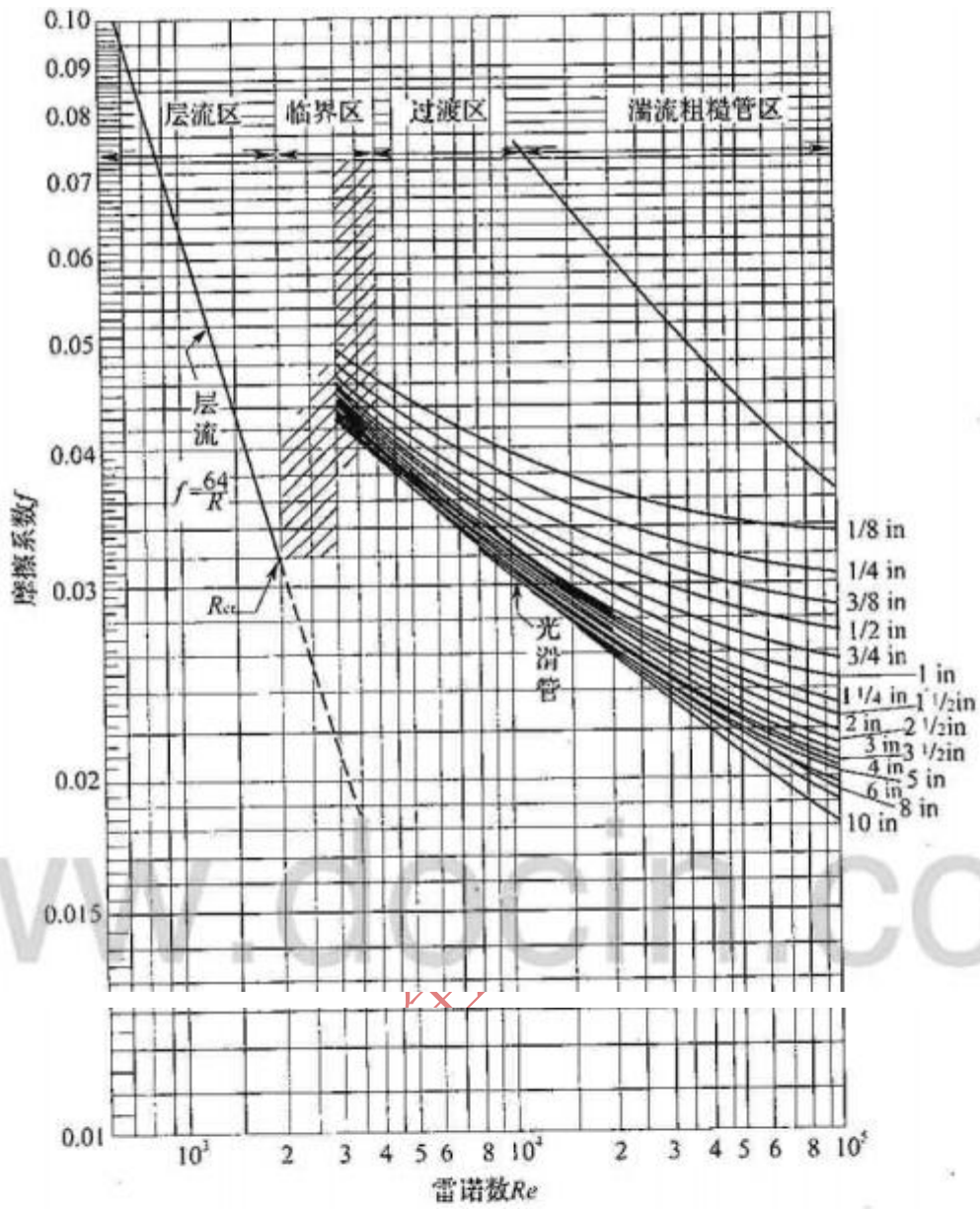
图 8 钢管莫迪图 ( Re \leq 10^5 )
