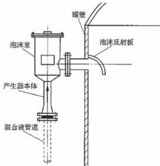
图3 立式泡沫产生器安装示意
