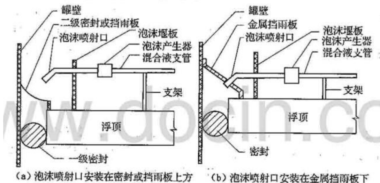
图 6 泡沫喷射口在浮顶上的安装方式
