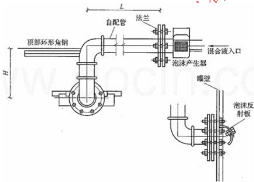
图4 横式泡沫产生器安装示意
