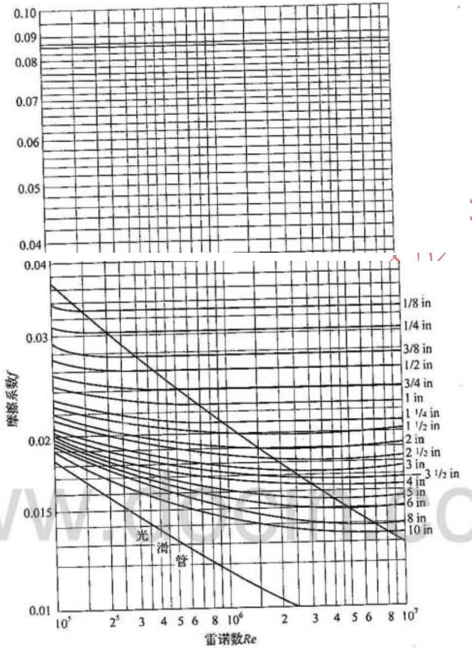
图 9 钢管莫迪图 ( Re \geq 10^5 )
