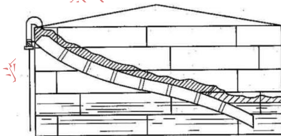
图 5 泡沫溜槽
