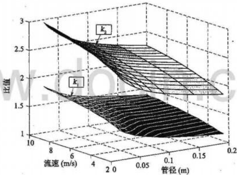
图 7 水力计算公式对比
